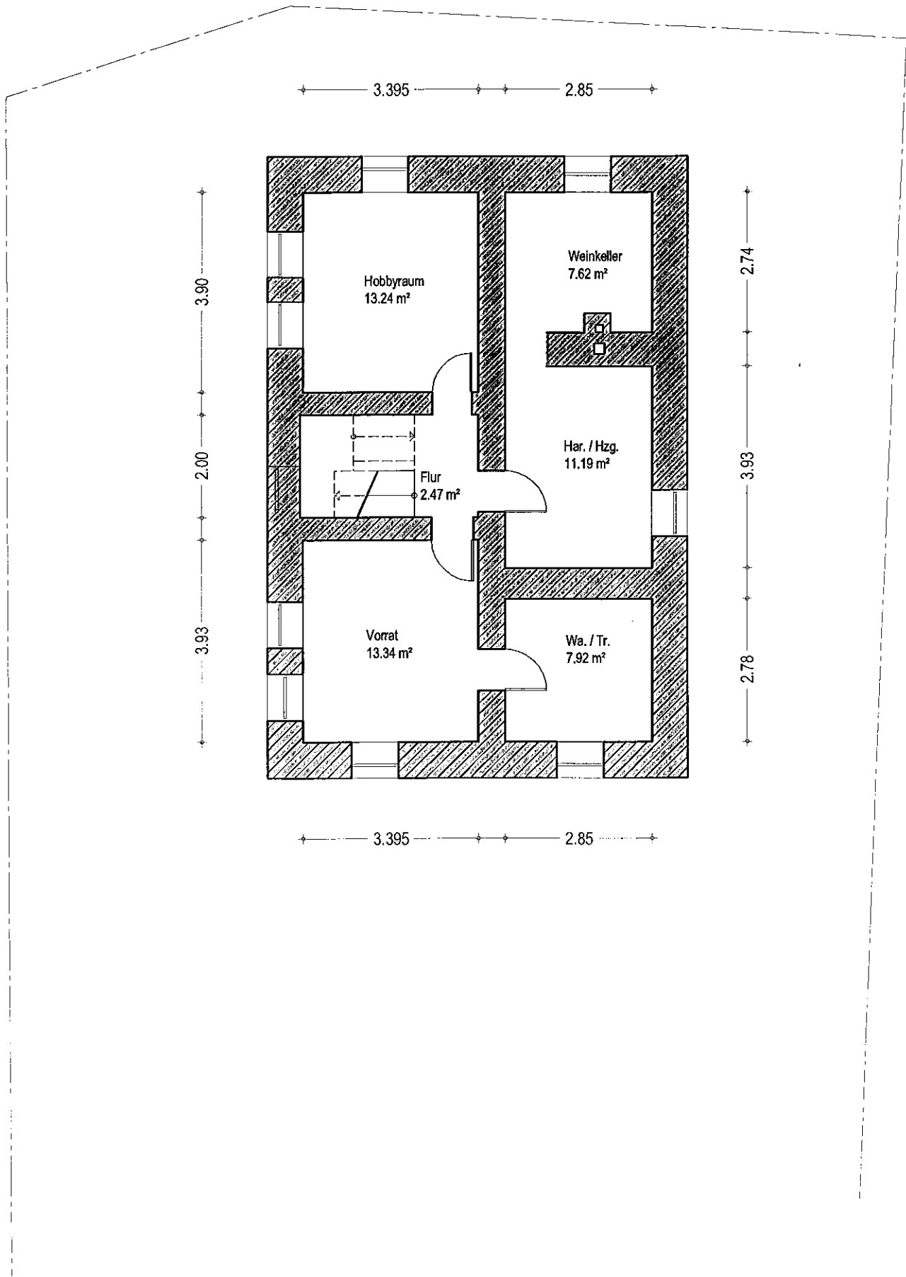
GRUNDRISS UNTERGESCHOSS
